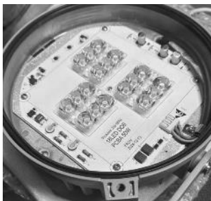
Vaihdeettava LED-moduuli
